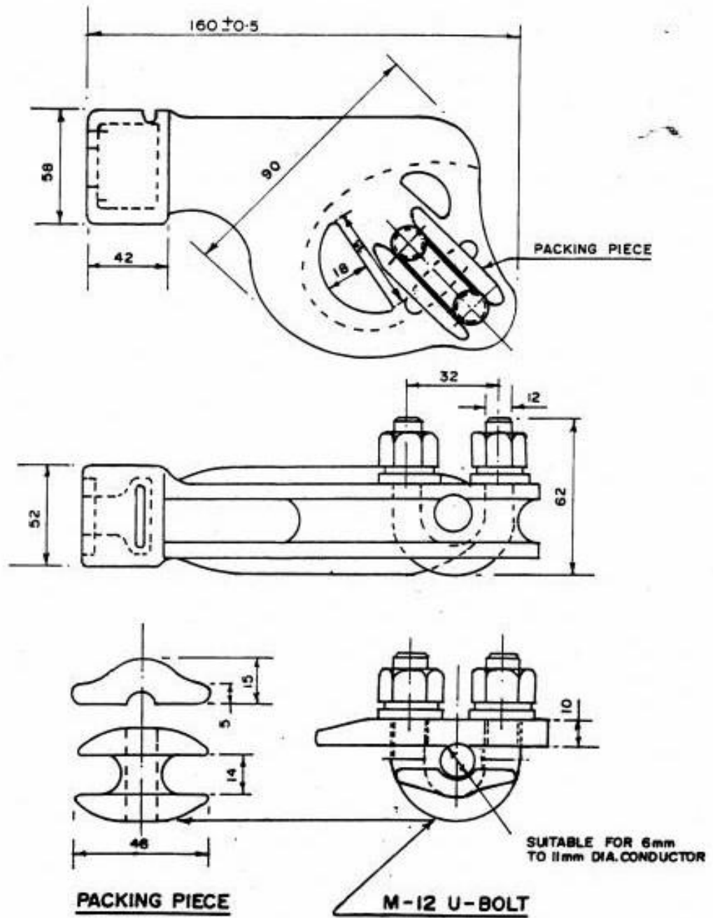
चित्र- 10. बॉल और सॉकेट प्रकार के विद्युत् रोधक के लिए एक की-विकृति (स्ट्रेन) क्लैम्प FIG. 10 - 11KV. STRAIN CLAMP FOR BALL AND SOCKET TYPE INSULATOR.
