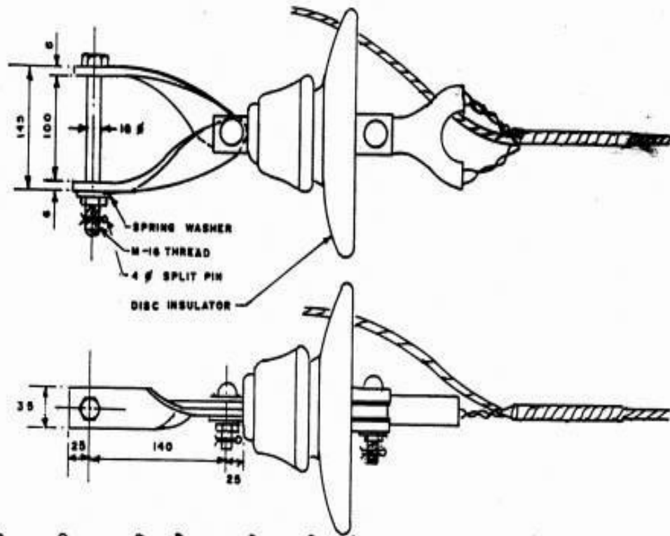
चित्र ५. टी. एण्ड सी. स्ट्रेन इन्सुलेटर एसेम्बली घुमावदार आकार फिटिंग सहित FIG.5. T & C STRAIN INSULATOR ASSEMBLY WITH HELICALLY FORMED FITTING
